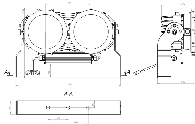
Рисунок 2. Габаритный чертеж.
